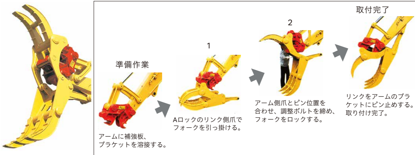
■ロッキーフォーク
